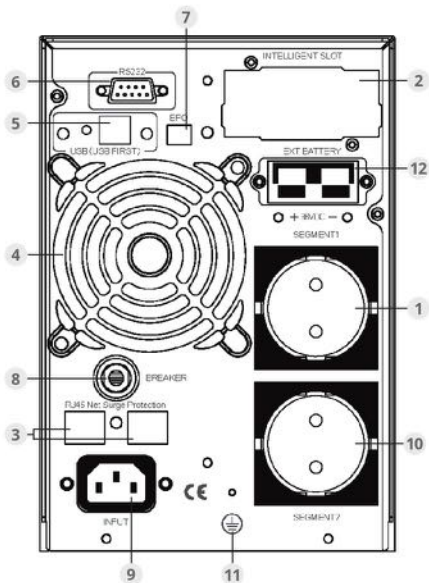
Рис. 2: Вид сзади: ИБП ИМПУЛЬС СТАЙЕР11-1 (1 кВА)
