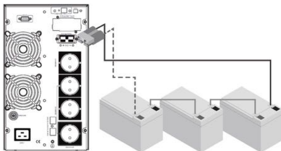
Рисунок 6. Подключение внешних АКБ к ИБП
