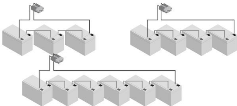
Рисунок 5. Подготовка внешних АКБ
