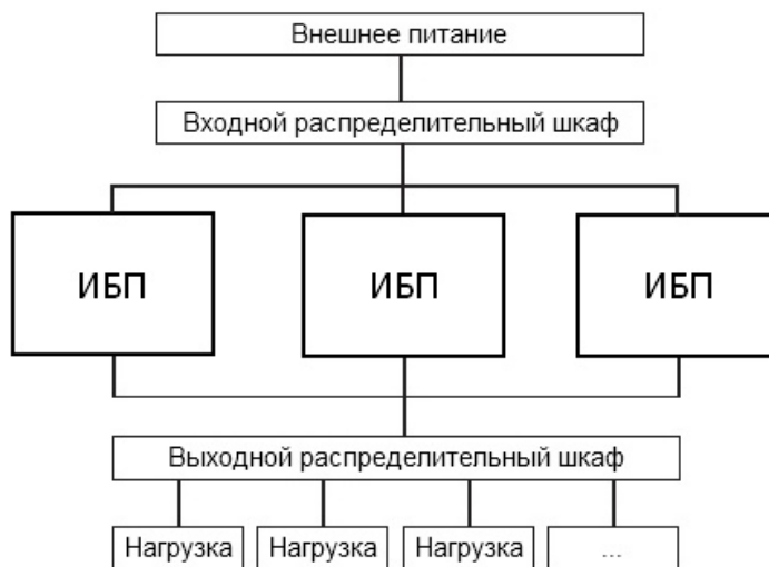
Структурная схема параллельной системы
