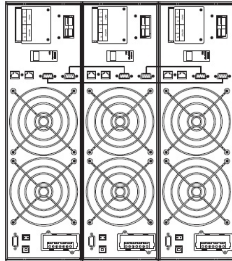
Параллельная система из трех ИБП
