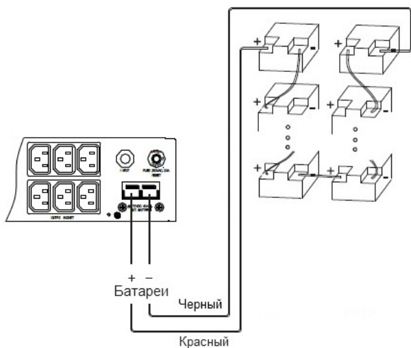
Схема подключения внешних батарей для ИБП 1кВА - 3кВА
